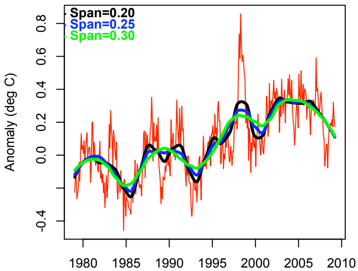
RSS Global Temp
